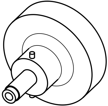
Positionierhülse für Handcrimpzange 09 99 000 0501 Locator for hand crimp tool 09 99 000 0501
